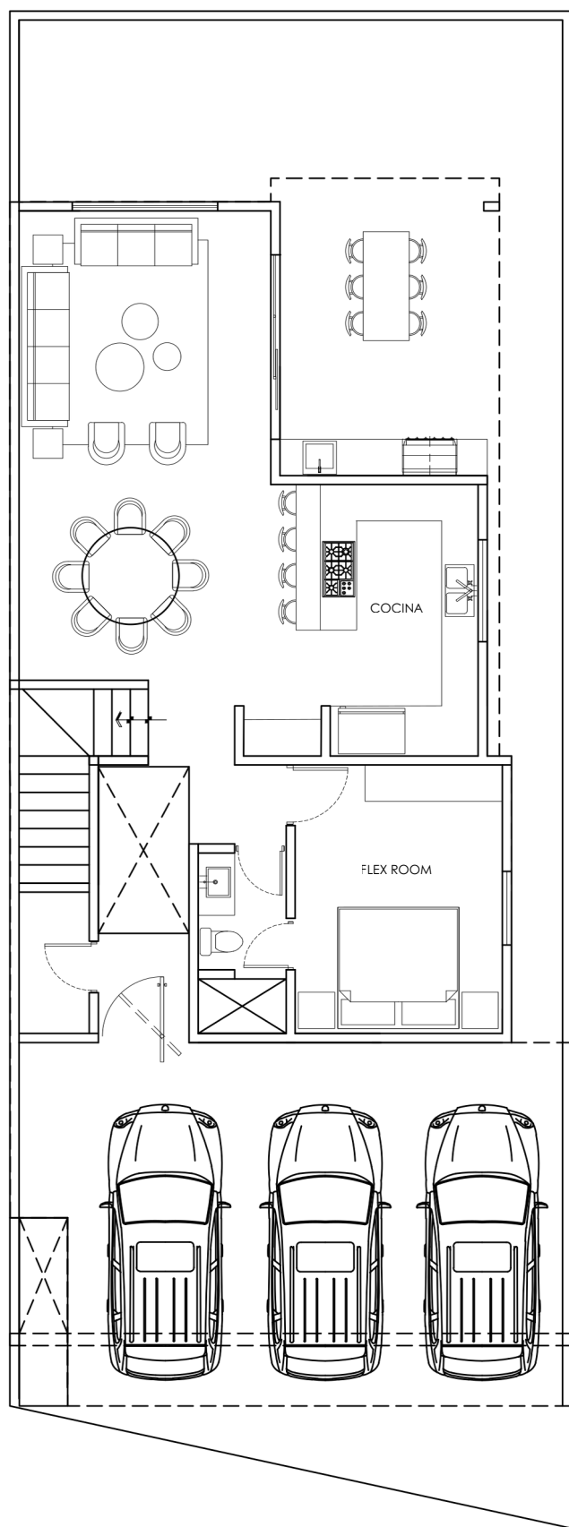
PLANTA BAJA
