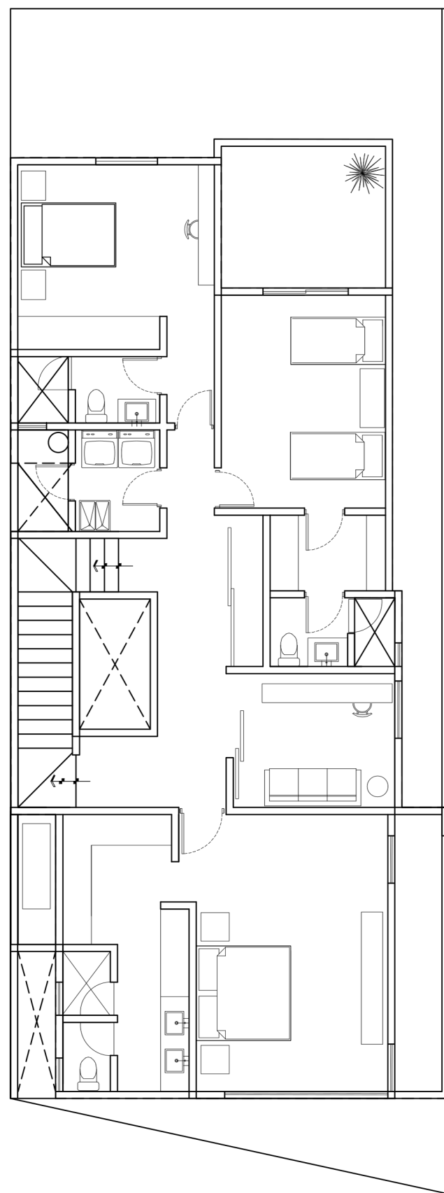
PLANTA ALTA
